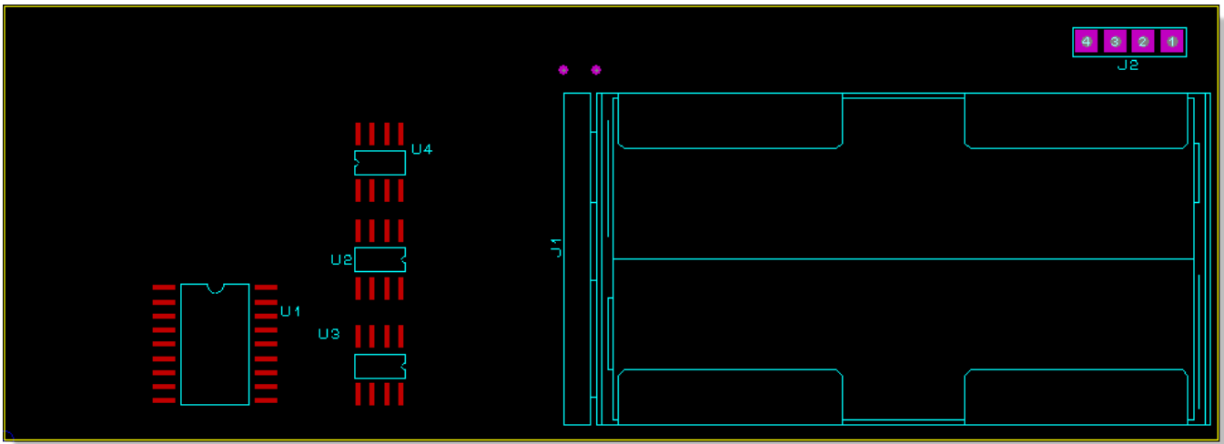
dsPIC33board so far...
