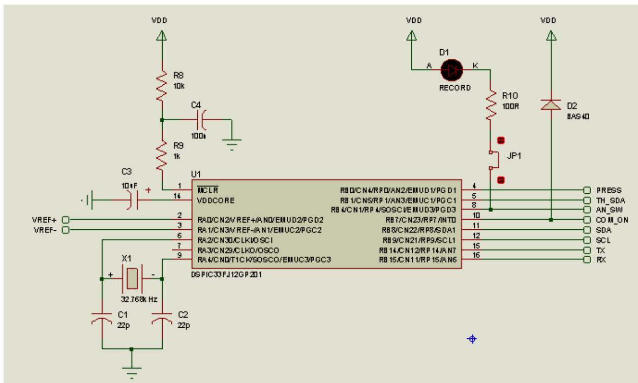
dsPIC33 Circuit section
